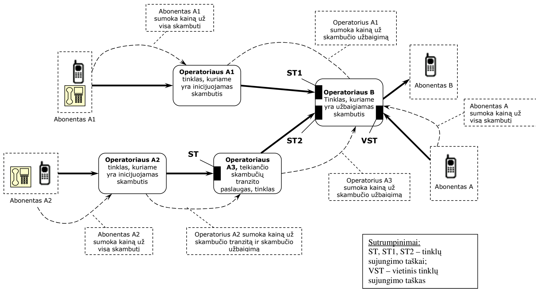
3 paveikslas. Individualių viešųjų telefono ryšio tinklų sujungimas.
