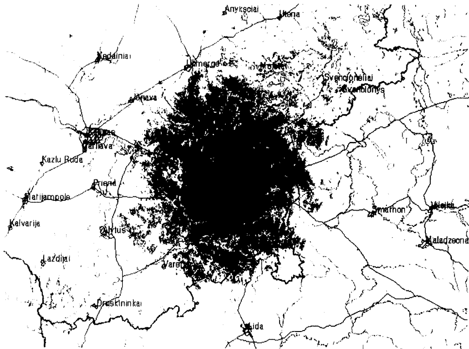
1 pav. Teorinė pirmojo siuntimo tinklo aprėpties zona – Vilnius.
