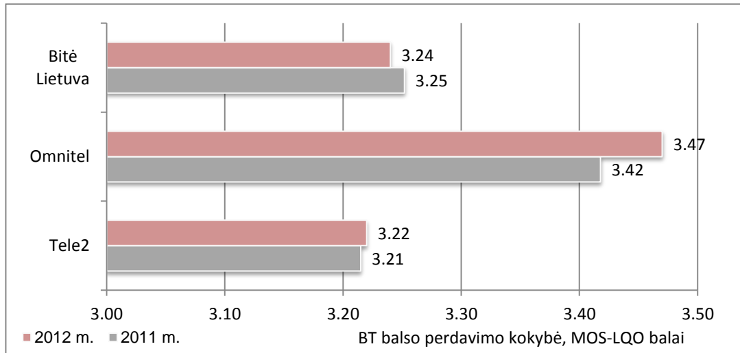
23 pav. Vidutinės BT balso perdavimo kokybės vertės 2011 ir 2012 metais
