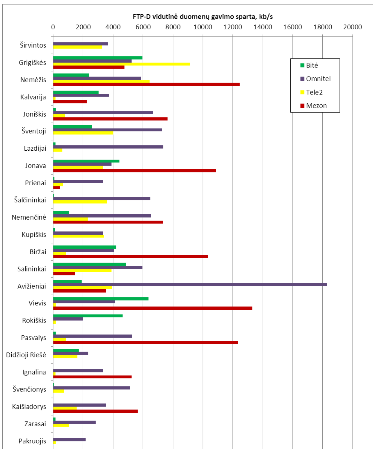
17 pav. FTP-D vidutinės duomenų gavimo spartos vertės įvairiuose Lietuvos miestuose (tęsinys).
