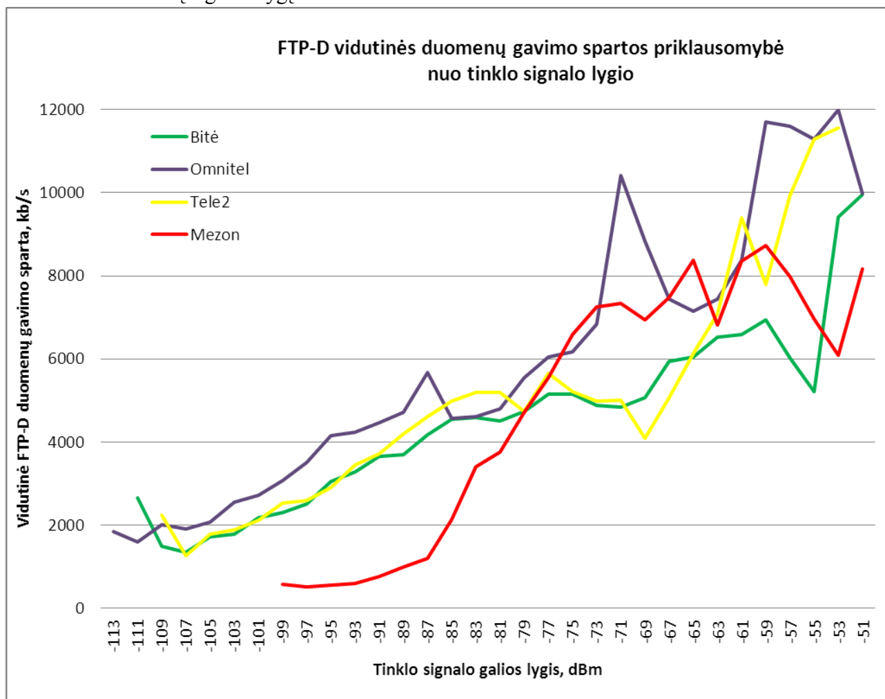
19 pav. FTP-D duomenų gavimo spartos priklausomybė nuo radijo ryšio signalo galios lygio atliekant bandymus
