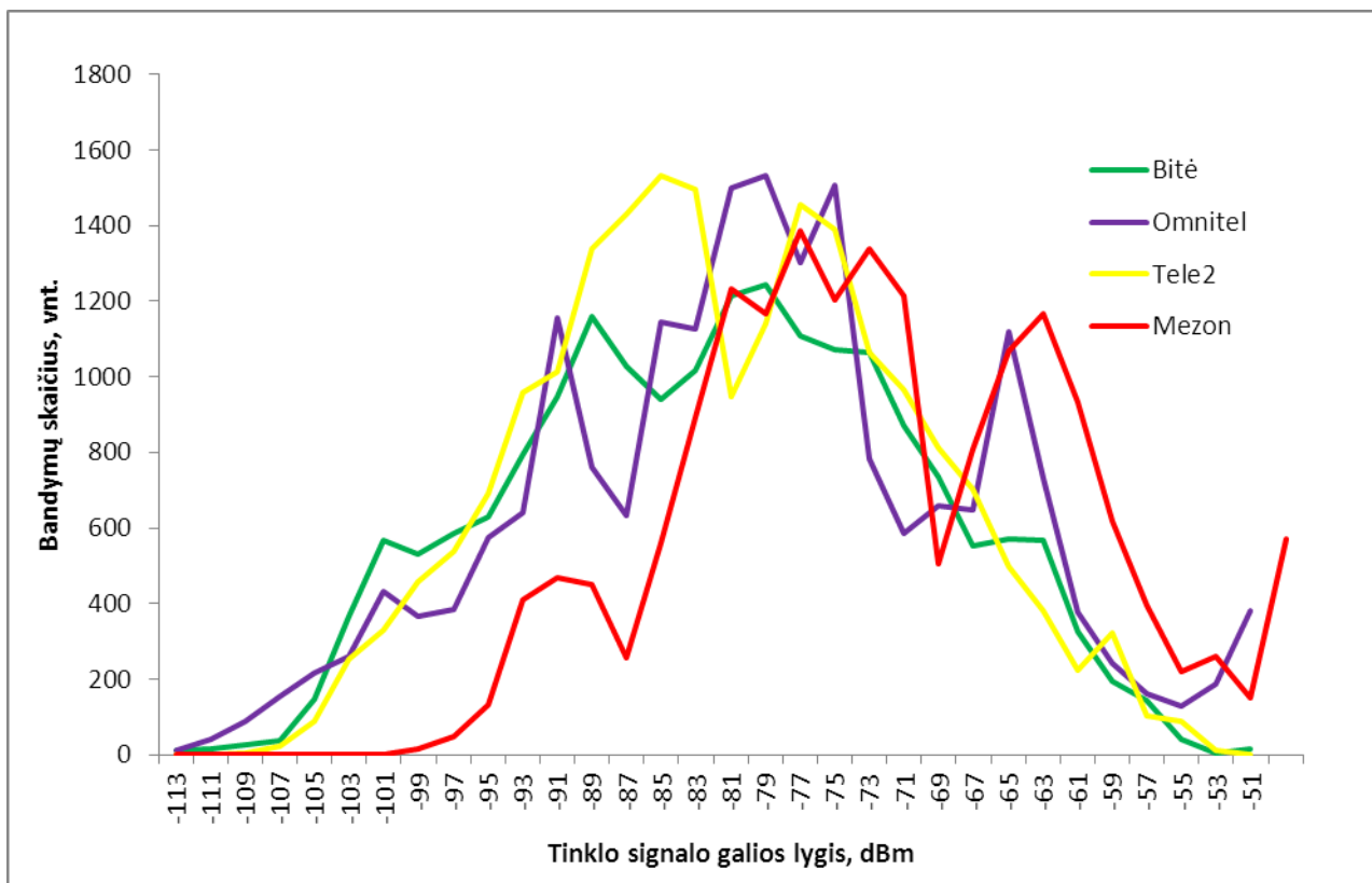
18 pav. Tinklo radijo ryšio signalo galios lygio verčių pasiskirstymas atliekant bandymus
